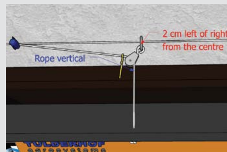
Plaatsen van katrol/klemmen en knopen van het touw
