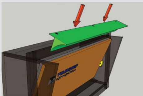
Plaats het kunststof profiel op de klep
