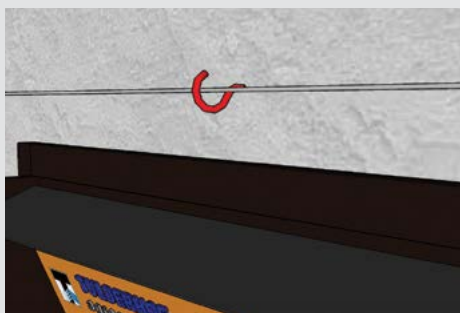
Schoefhaken plaatsen 2 cm links of rechts van het midden, trekdraad door schroefhaak
